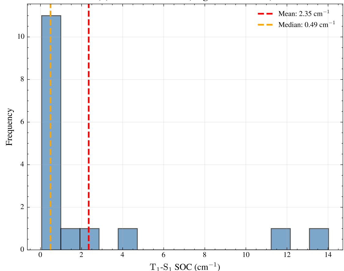
(d) SOC Distribution (Organic Molecules)
